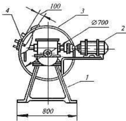
1 - станина; 2 - двигатель; 3 - барабан; 4 - полка барабана
