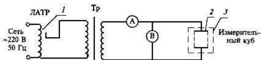
Рисунок 15 - Измерительная схема
