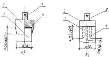
Схема приклеиваемых и анкерных захватов
