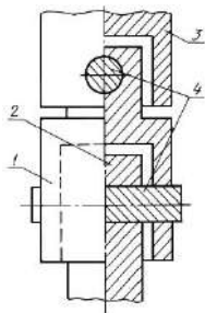
Схема шарнира Гука
