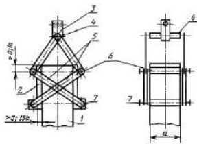
Схема самозажимного зажима
