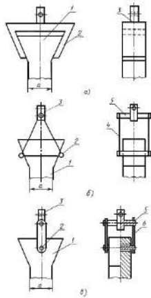
Схема захватов для образца с галтелями
